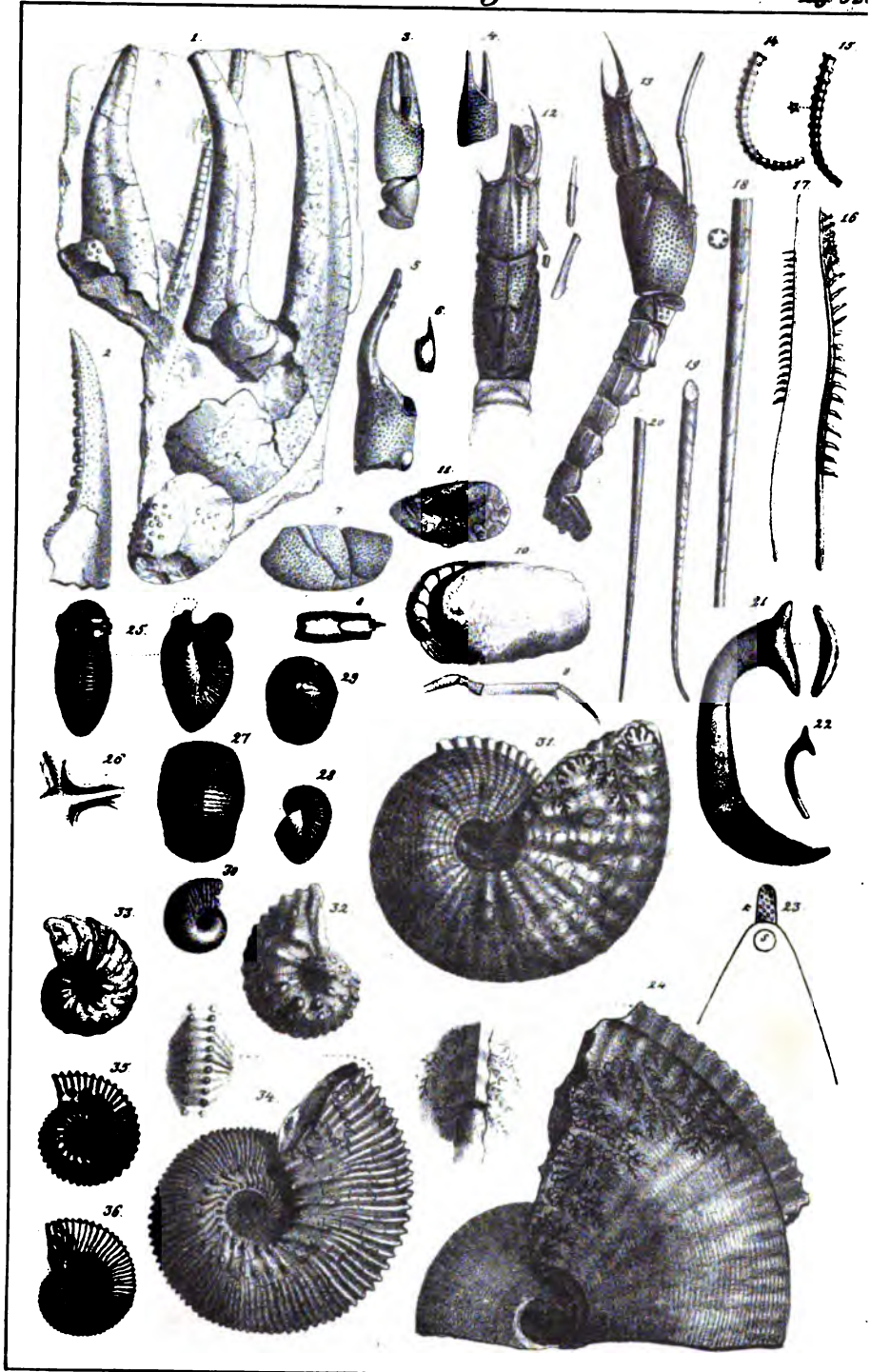
Quenstedt, Jura.
